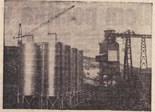
Prekladalna postaja za cement, kakršno je zgradil Itas Kočevje pri hidroelektrarni Bajina Bašta.
