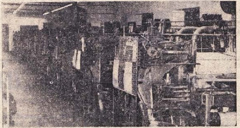
Takole je v Novoteksovi tkalnici, odkar so jo opremili z enotnimi stroji, ki so izdelek domače tovarne Tekstilstroj iz Zagreba
