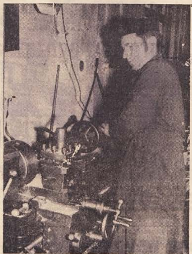
Tone Zobarič struži v »METALU« (Jesenice na Dol.) kovinske dele za električne vtičake in pritezne vijake.
