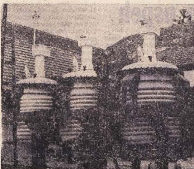
Trije reaktorji po 3000 litrov čakajo. V kratkem jih bodo predali naročniku, tovarni »IPLAS« v Koprju. Takih in manjših reaktorjev bodo v podjetju »Kemo-oprema« v Trebnjem letos izdelali še več
