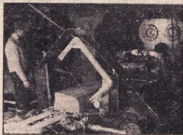
Pogon nove »vakuum stiskalnice«. — Pretekli teden so v strojnem oddelku zaloške opekarne montirali pod vodstvom Pavleta Dolenca, strokovnjaka iz Litostroja, novo stiskalnico za opeko. Napravo so takoj tudi preizkusili; z delom vred bo veljala kakih 12 milijonov dinarjev. Več o opekarni Zalog berite na 5. strani današnje številke!
