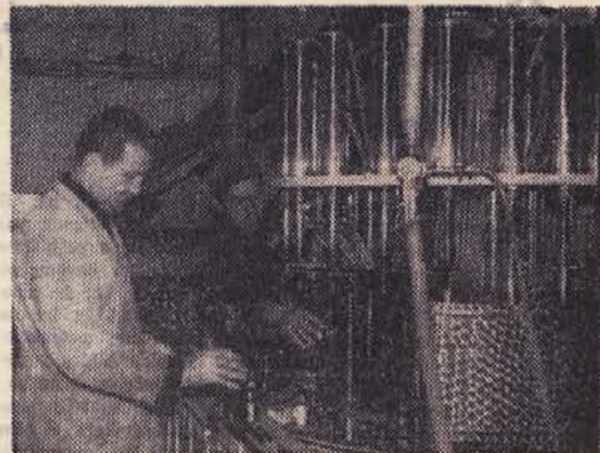
Na sliki vidite najsodobnejšo polnilno napravo, ki steklenice opere, napolni z vinom, začepi in etiketira. Stroj je v Italiji kupilo podjetje »Vino« in Brežice in je edini te vrste v Jugoslaviji. Brez dvoma bo veliko pripomogel k buteljiranju vin, za kar je v naši potrošnji vin že skrajni čas
