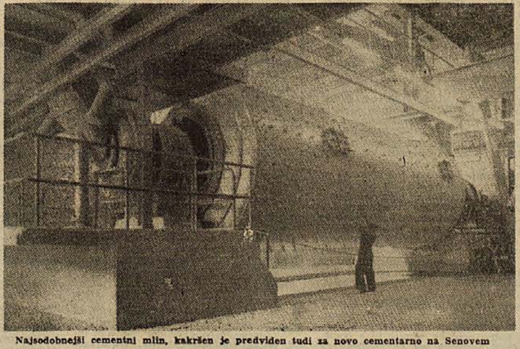
Najsodobnejši cementni mlin, kakršen je predviden tudi za novo cementarno na Senovem
