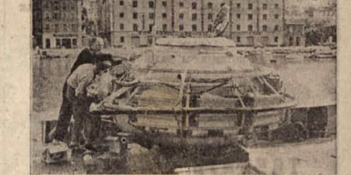
V malem zalivu v Nici na francoski obali so se dni radevedneži ogledovali čudno vozilo, ki ga je skonstruiral Francouz Cousteau. Gre za pomorski letični krožnik, ki se s precejšnjo naglico lahko giblje 400 m globoko v morju. Vozilo je opremljeno s močnimi reflektorji in s posebnimi jeklenimi šapami ter je namenjeno podmorskim raziskovanjem.
