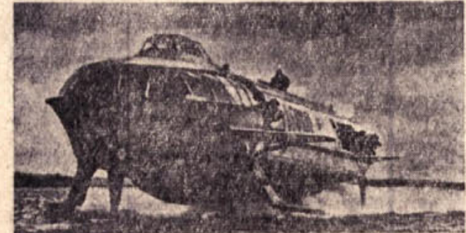
Minulo jesen so v zavodu Rdeče Sormovo izdelali hidrobuss na krilih. Dali so mu ime »Meteor«. Od tedaj je uspešno pre-stal vse preizkušnje in prehaja zdaj v redni promet. Ima pro-stora za 150 pomikov, izdelan je ves iz duruminija, doseže pa hitrost do 80 km na uro. V istem zavodu so že napravili načrte za nov, še večji hidrobuss, ki bo lahko vzel na krov 200 pomikov, razvil pa bo hitrost 100 km na uro. Vozil bo po Azovskem in Crnem morju, kjer so delali poskuse tudi z »Meteorjem« (na sliki).
