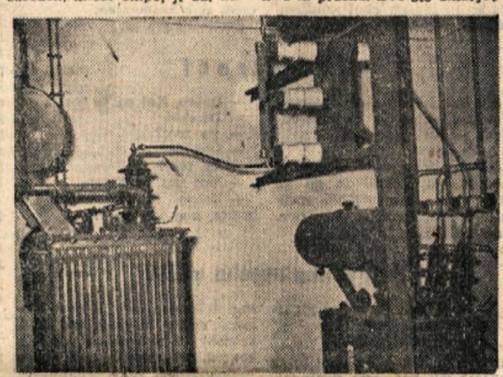
— To je naša peterzenka, so nam rekli na RTP Bršljin in dodan-ta naprava kompenzira zemeljskostične toke, kadar so nevlhte.
