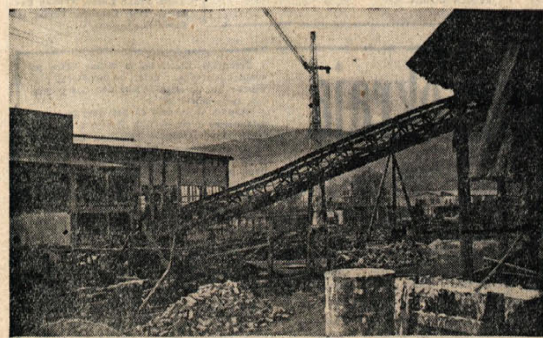
Ena izmed letošnjih velikih delovnih zmag naših kolektivov: v soboto bodo v Straži zaključili gradbena dela nove tovarne podjetja NOVOLES, ki je zrasla od letošnjega aprila do konca novembra; več o tem preberite na strani, ki smo jo v današnji številki namenili kolektivu NOVOLESA
