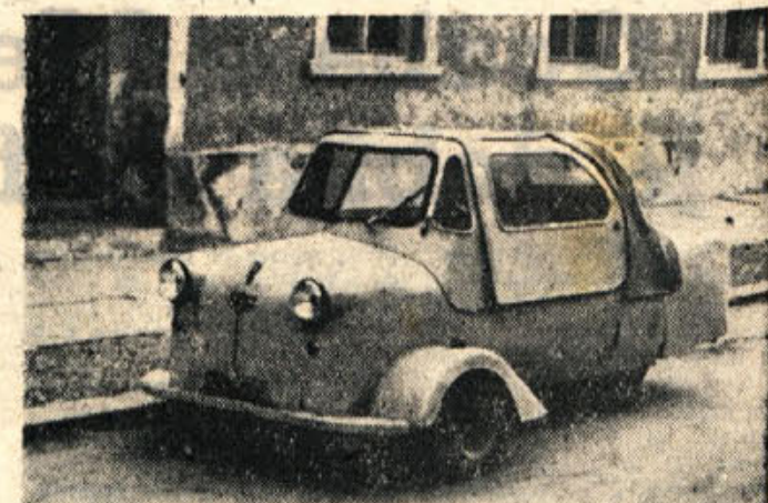
Ne navaden obisk v Brežicah: svojevrstno vozilo — recimo mu kar avtomobil — na 3 kolesih, s katerim je prišel inozemski turist v Spod. Posavje, je vzbudilo pred kratkim precej zanimanja med brežiško mladino
