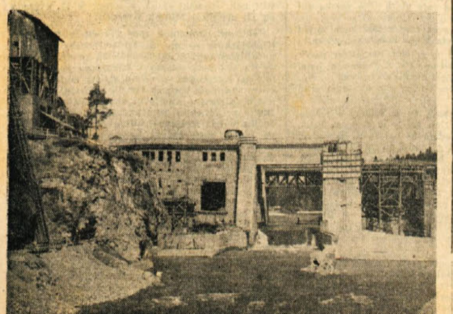
Hidrocentrala v Medvodah, ki bo začela delati prihodnje leto
