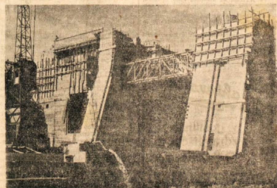
Med velikimi pelletke, ki so ponos naših ustvarjalcev socializma, je tudi hidrocentrala v Medvodah. Za pregrado, ki jo vidimo na sliki, se bo zbralo umetno jezovo, iz turbin v centrali pa se bo pretekala v industrijo in domove električna energija.
