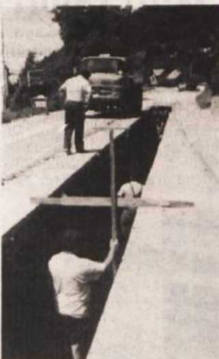
CEVI NISO POŽIRALE VODE - V teh dneh bi po napovedih Šmarška ulica v Sevnici že morala biti spet odprta za promet, prebivalci ob njej pa ob večjem deževju bolj mirni. Ves pretekli teden so namreč delavci sevniske komunale urejali razbremenilno kanalizacijsko omrežje. Kot nam je povedal vodja gradbišča, se je naseleje nad ulico vse bolj širil, česar presek pod cesto vgrajenih cevi ni več vzdržal. Tako cevi ob nevihtah niso več požirale dodatnih količin vode, ki je tekla po ulici in že večkrat zalila kletne prostore sosednje gostilne. Zaradi tridnevne popolne zapore je bil promet namesto na most preusmerjen po drugi strani železnice na prehod nekoliko nižje. (Foto: B. D. G.)
