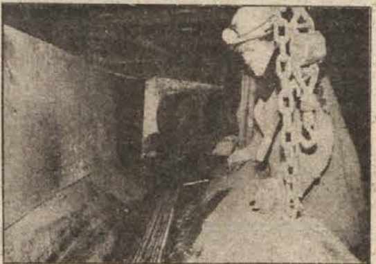
TRANSPORTNI TRAK — Za delovanje gumijastega transportnega traku, ki iz čelnih kopov prevaža premog v zbirališče, skrbi tudi vzdrževalec, strojni ključavničar Srečko Švajger. Z vsemi delovišči je povezan s posebnim signalnim sistemom, preko katerega kopači in transportni delavci dobivajo sporočila in navodila.
