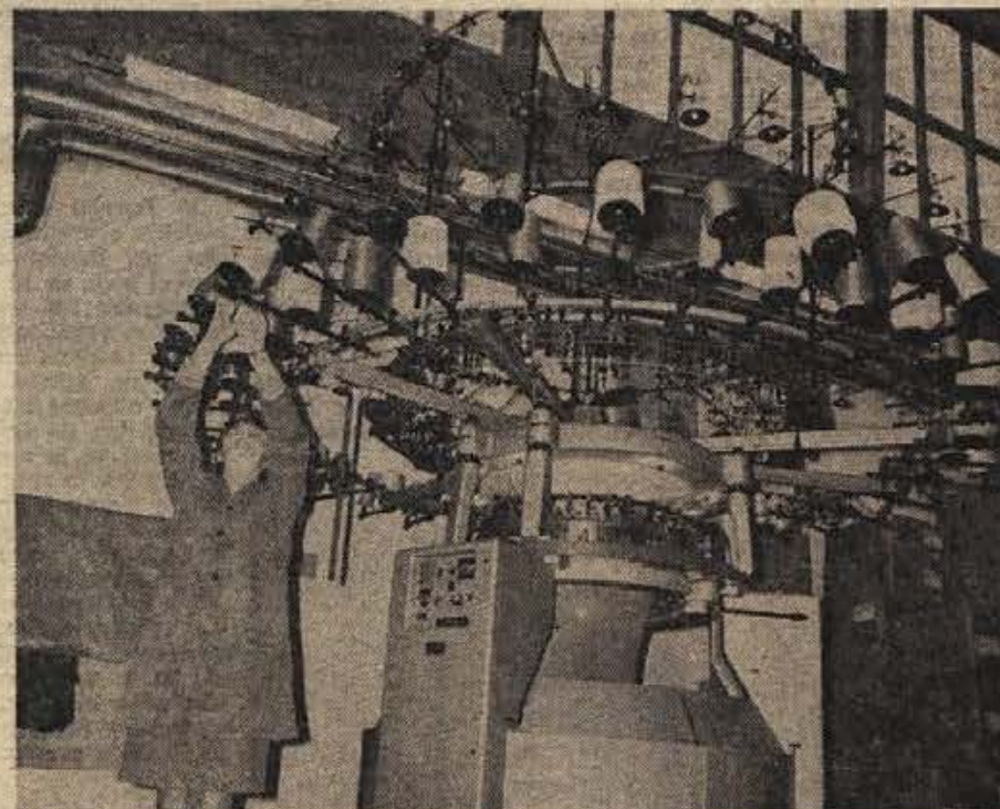
Zadaji krik mode: stroj za pletenje moških in ženskih tkanin
